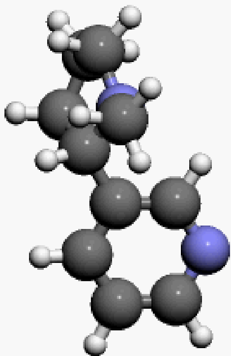
โมเลกุลของสารนิโคติน
